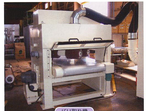
バリ取り機
